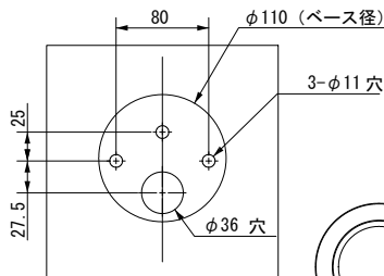
取付対象板 穴寸法図
