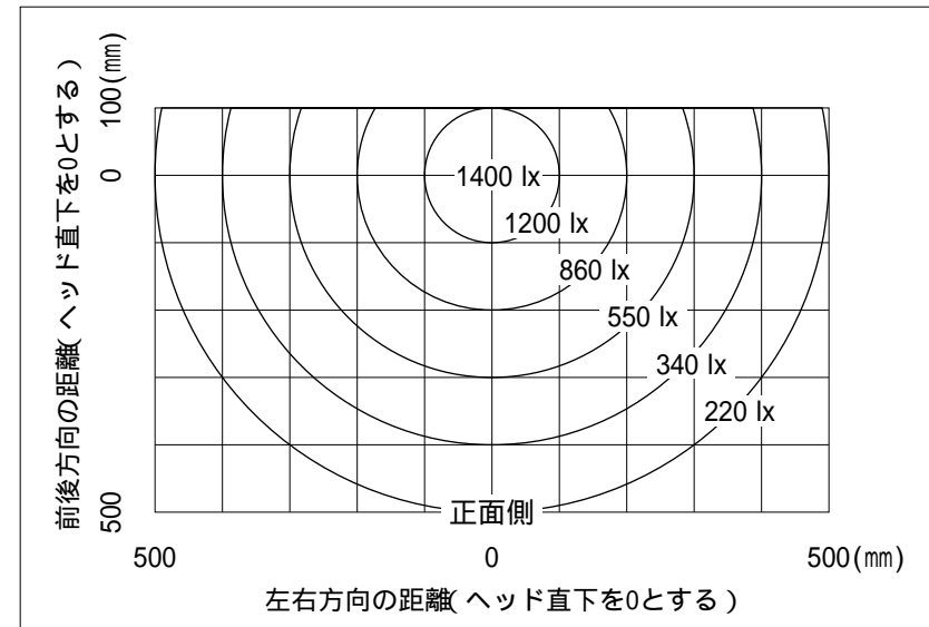
照度分布図
