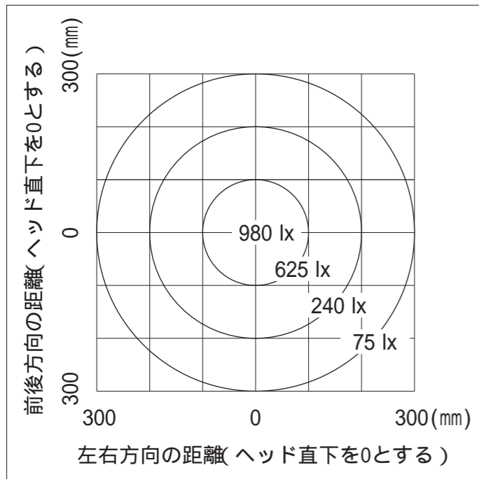
照度分布図
