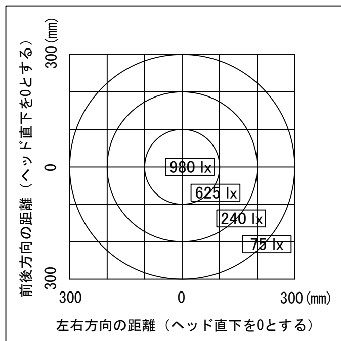
照度分布図
