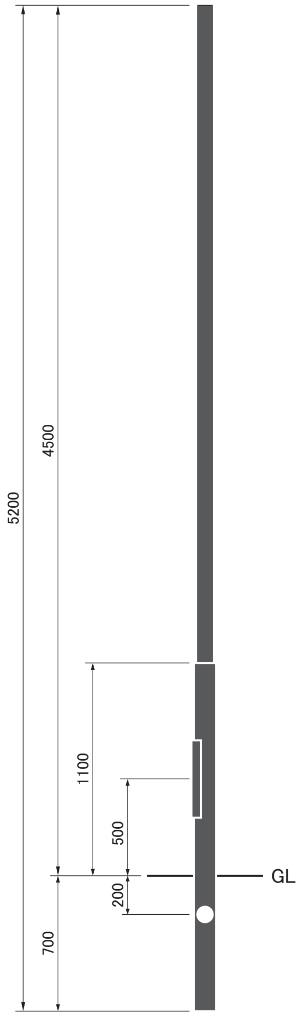
ポール型式: LPA45-425 溶融亜鉛メッキ仕上げ
