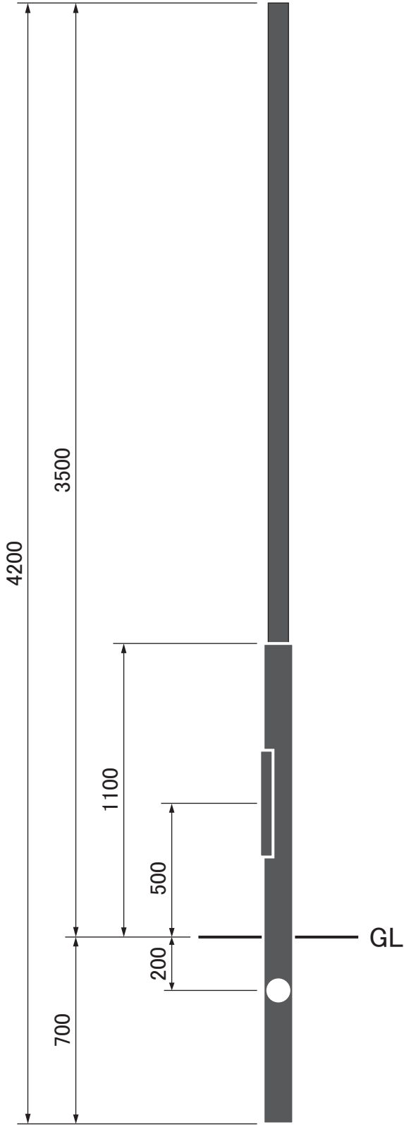
ポール型式: LPA35-425 溶融亜鉛メッキ仕上げ
